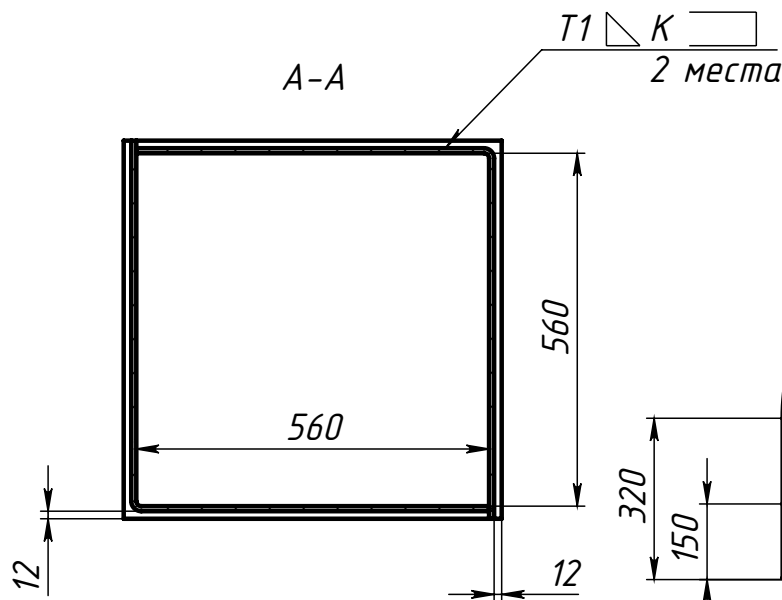
Поз.3 (Ложемент)
