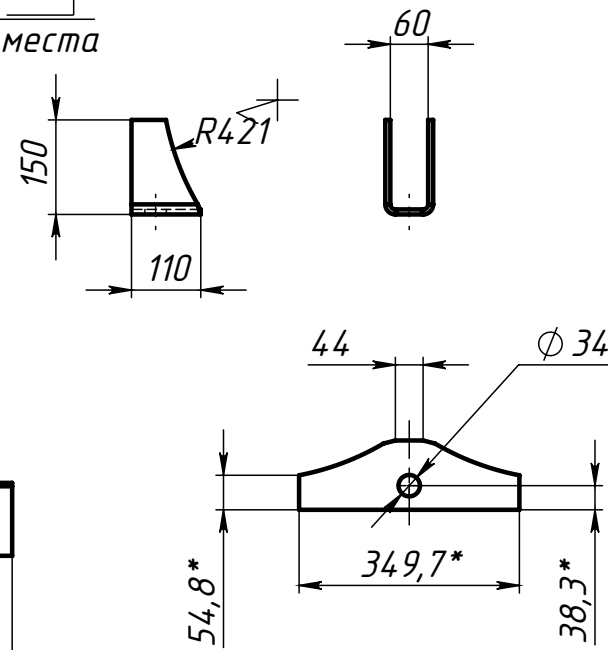
Поз.4 (Ушко)
