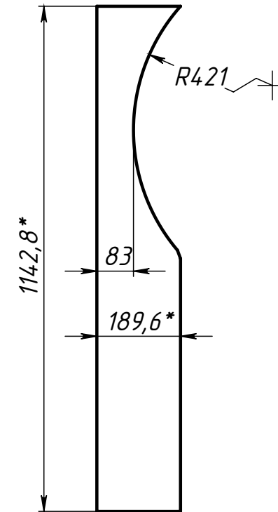
Поз.2 (Корпус) развертка
