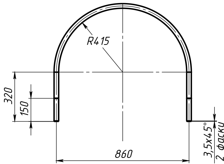
Поз.6 (Упор)
