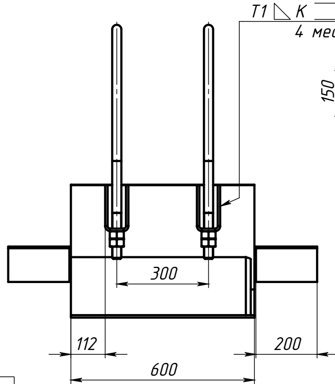
Поз.5 (Хомут) 1 : 15
