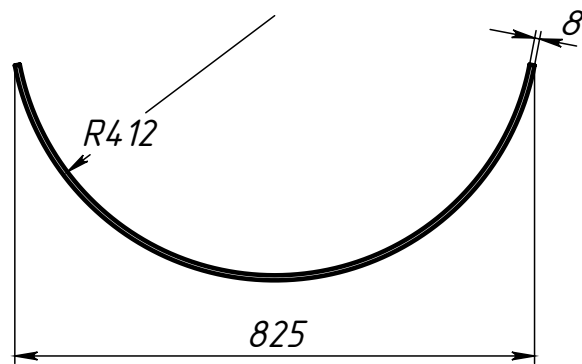
Поз.3 (Ложемент)
